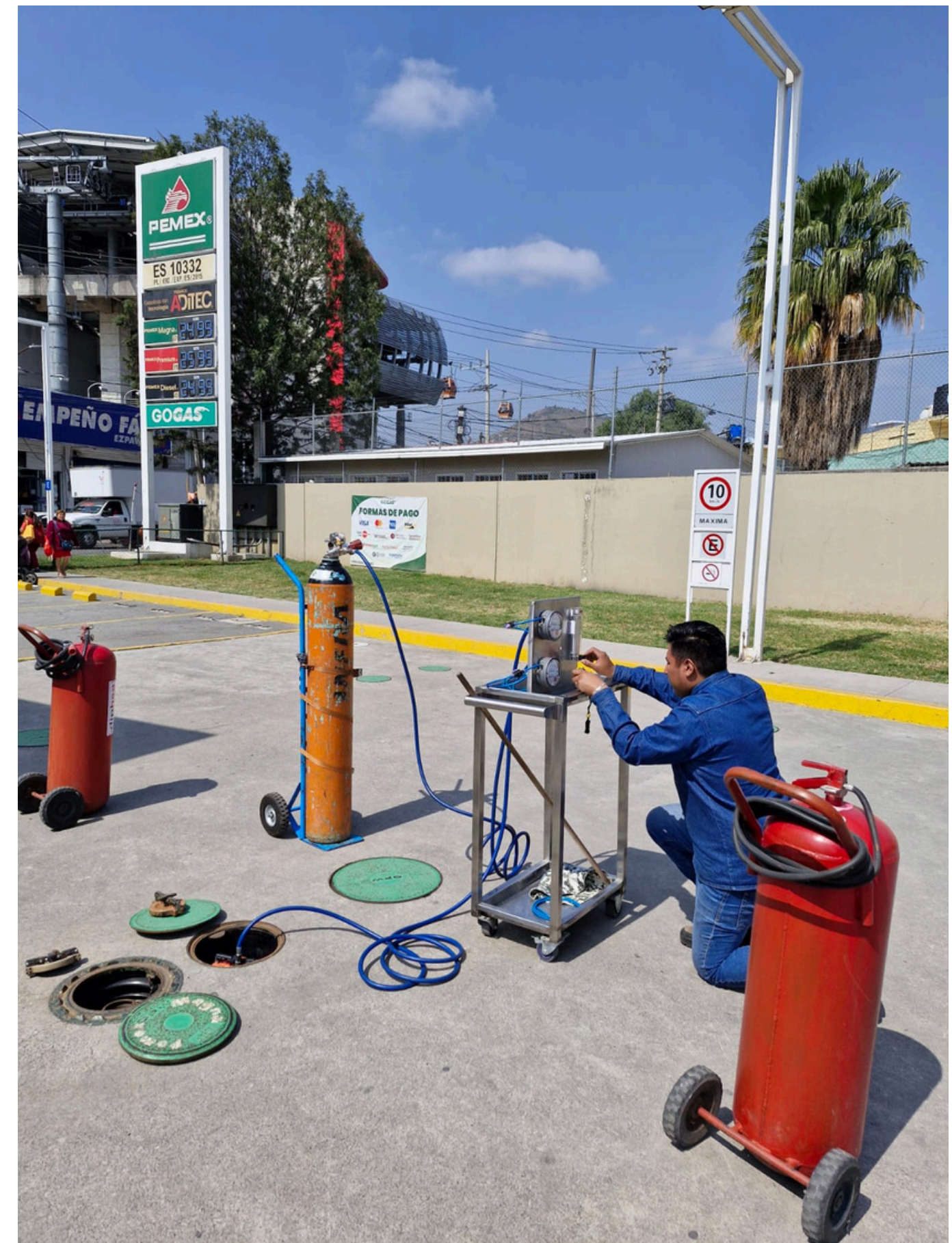
Prueba - Determinación de la presión estática en 5 y 2 pca
